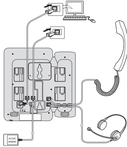
• 그림1 : 1000i 시리즈 전화기 연결
