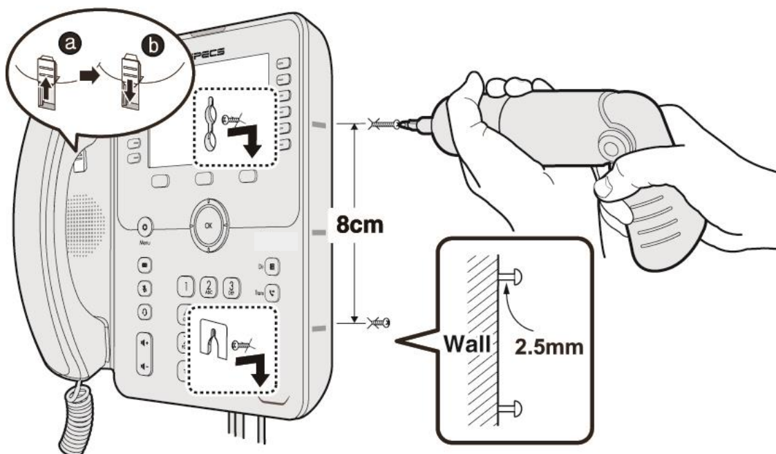
그림 1.6: 벽걸이 설치
