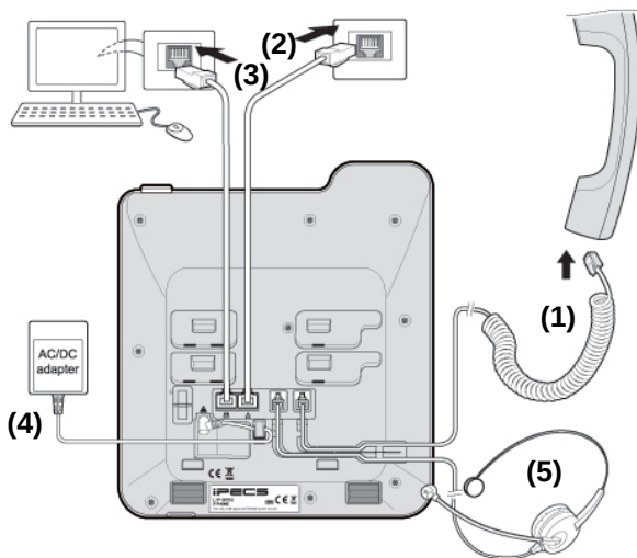
그림 3 LIP-9008/LIP-9008G 연결
