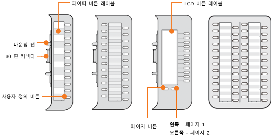
그림 4 LIP-9012 DSS, LIP-9024 DSS, LIP-9024 LSS, LIP-9048 DSS
