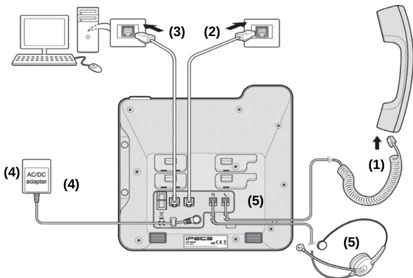
그림 9 LIP-9000시리즈 연결
