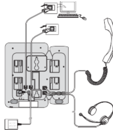
그림1: 1000i 시리즈 전화기 연결
